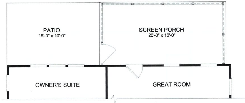
OPTIONAL SCREEN PORCH
